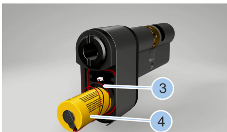
Abb. 149: Batterie einsetzen
