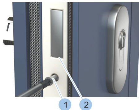
Abb. 32: Stulpschraube anziehen
